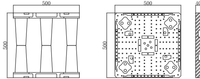
儲集框架主體 構造圖
